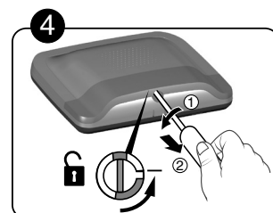
4 Déverrouillez le boîtier.
