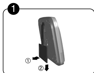
1 Séparer le support mural du TYDOM 2.0.
