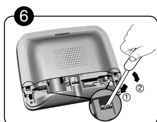
6 A l'aide d'un tournevis, soulevez les 2 clips du capot supérieur.
