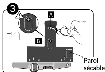
3 Fixez le support mural à l'aide de 2 vis Ø 4 mm Max. en utilisant les trous A et B. N'utilisez pas de visseuse pour visser la vis repérée B.
